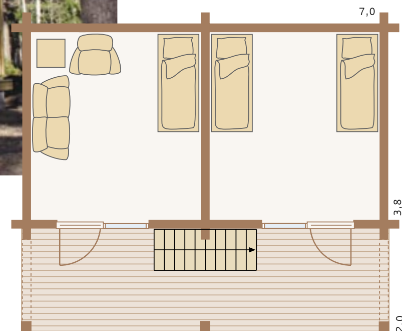
1:75 ALAKERTA
