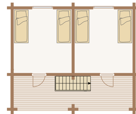
1:125 YLÄKERTA
